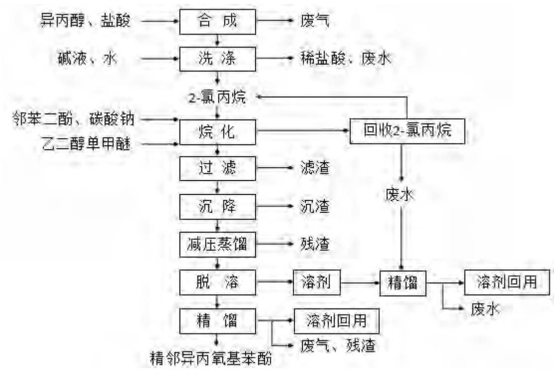
图 3-1 工艺流程及产污环节
