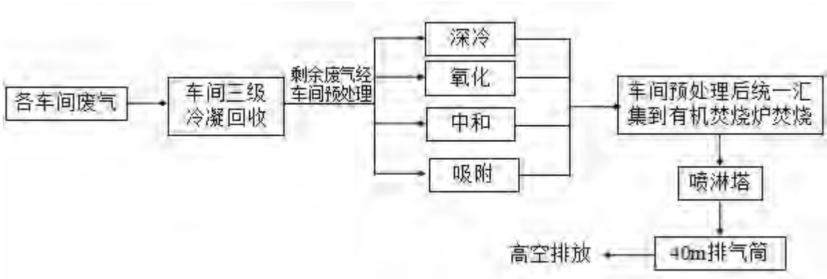
图 4-3 废气工艺流程图
